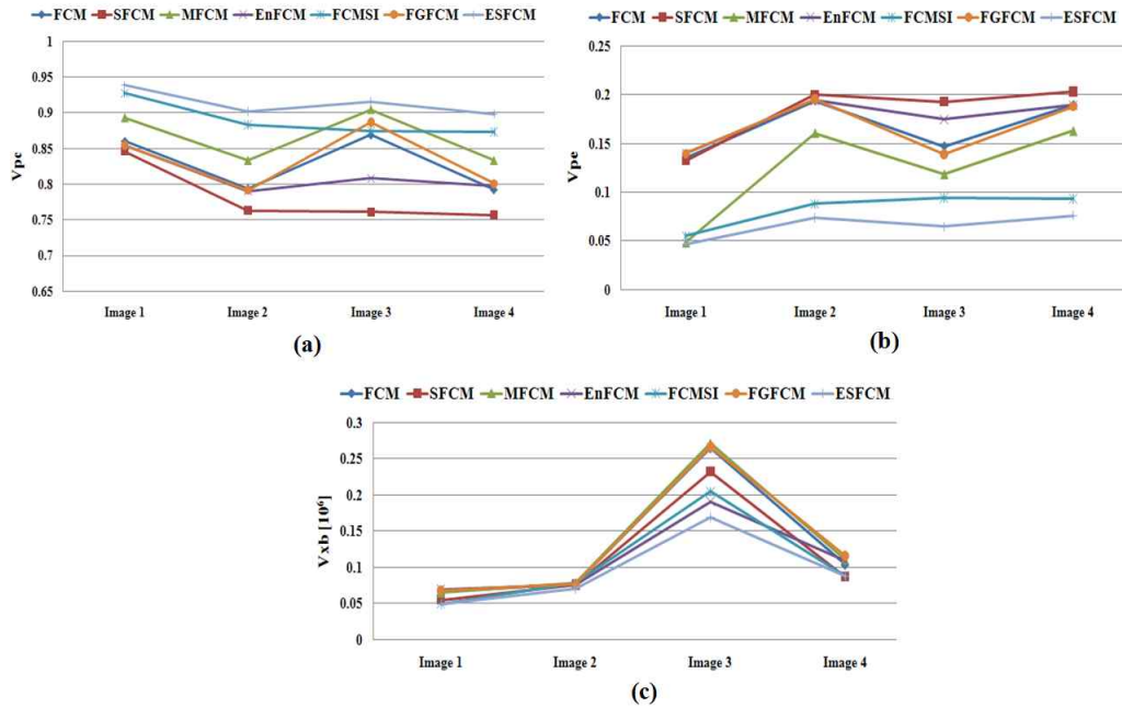
그림 2. c=4 를 가지고 제안한 ESFCM 알고리즘과 기존의 FCM 기반 알고리즘의 클러스터링 성능. (a) V_{pc} , (b) V_{pe} , and (c) V_{xb} Fig. 2. Clustering performance between the proposed ESFCM algorithm and conventional FCM based algorithms with c=4 . (a) V_{pc} , (b) V_{pe} , and (c) V_{xb}
