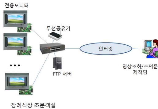
그림 4. 프로토타입 시스템 구현을 위한 구성도 Fig. 4. Structure for implementing Prototype System
