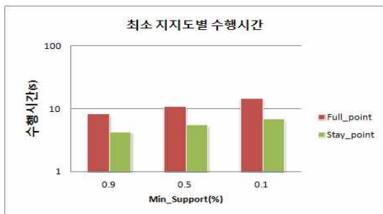
그림 6. 최소 지지도별 수행시간 Fig. 6. Execution time
