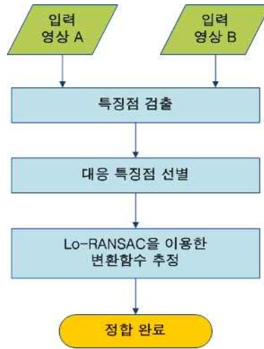
그림 1. 제안하는 영상정합 기법의 전체 구조 Fig. 1. Overall structure of the proposed image registration method
