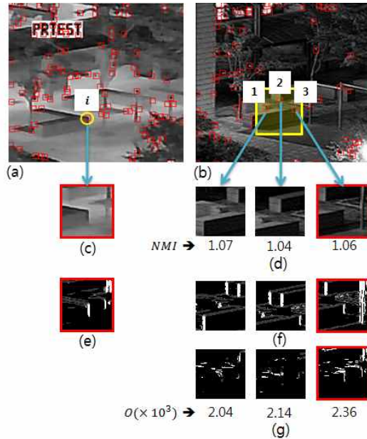
그림 4. 제안한 유사성 척도를 이용한 대응점 선별 과정. (a), (b) 적외선 및 가시광선 영상에서 추출된 특징점 (c), (d) 각 특징점의 패치 영상 (e), (f) 패치 영상의 기울기 방향 (g) <e>와 <f>간의 기울기 방향 각도 차이
