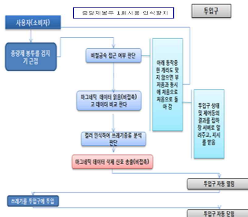
[그림6] 인식 시스템 흐름도 [fig.6] Flowchart of Recognition System
