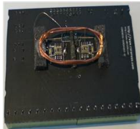
(b) 실험에 사용된 센서 (b)Sensor used in the experiments
