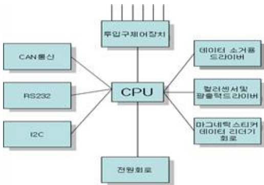
[그림4] 인식장치 블록도 [Fig.4] Recognition device block
