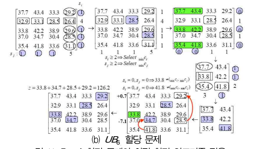
그림 11. 5×4 할당 문제의 최적 할당 알고리즘 적용
