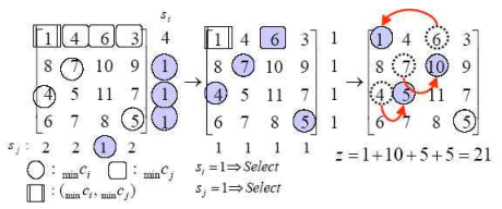
그림 4. A 문제의 최적 할당 알고리즘 적용 Fig. 4. OA Algorithm for A Problem
