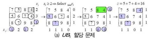
그림 9. 3×4 할당 문제의 최적 할당 알고리즘 적용
