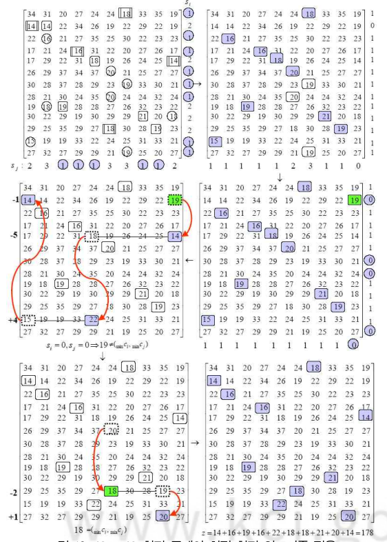
그림 12. 13×10 할당 문제의 최적 할당 알고리즘 적용
