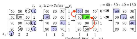
그림 10. 4×3 할당 문제의 최적 할당 알고리즘 적용
