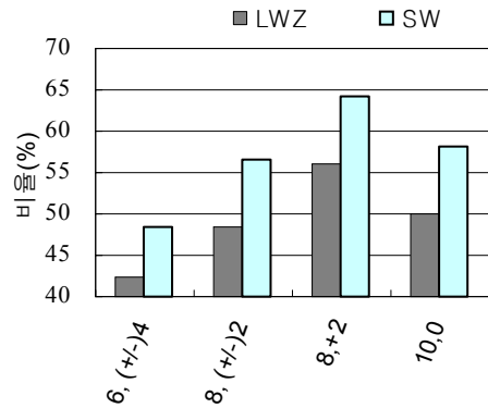
그림 13. 레지스터 필드, 즉시 필드 할당 비트 수에 따른 LWZ와 SW 명령어의 변환 비율 Fig. 13. The conversion ratio for the LWZ/SW instruction by the number of bits for register and immediate fields.
