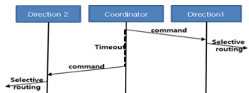
그림 6. 방향성 메시징의 메시지 방향 변경을 위한 메시지 시퀀스 Fig. 6. Message sequence for changing the message direction by Directed-Messaging
