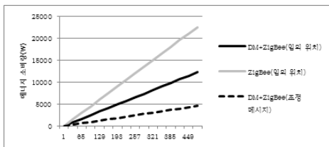
그림 10. 이벤트 발생 형태 정보에 따른 에너지 소비량 Fig. 10. Energy consumption according to information of event types
