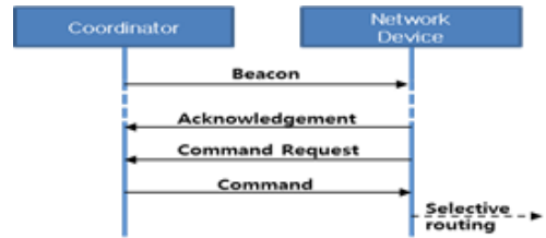
그림 5. 방향성 메시징 기법을 지원하는 수정된 지그비 비콘 모드 시퀀스 Fig. 5. Modified ZigBee beacon-mode sequence supporting Directed-Messaging
