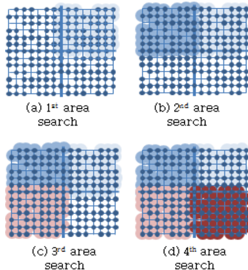
그림 2. 방향성 메시징의 소스노드 탐색 과정(5) Fig. 2. Searching for source node by Directed-Messaging(5)
