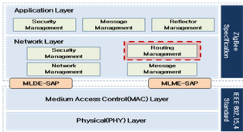
그림 1. 지그비/IEEE 802.15.4 스택 구조(2) Fig. 1. ZigBee/IEEE 802.15.4 Stack architecture(2)
