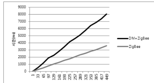
그림 11. 소스 노드 탐색 횟수에 따른 시간 소비량 Fig. 11. Time consumption according to the number of search
