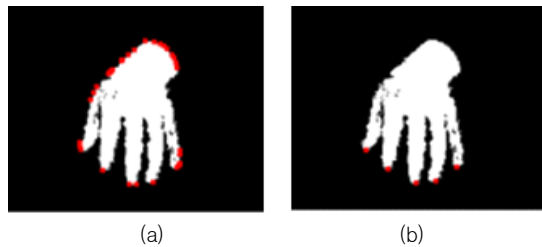
그림 8. (a) convex hull 검출 (b) 손가락 끝점 검출 Fig. 8. (a) convex hull detection (b) finger tip detection
