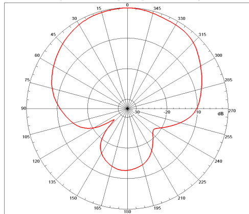
(a) H-plane
