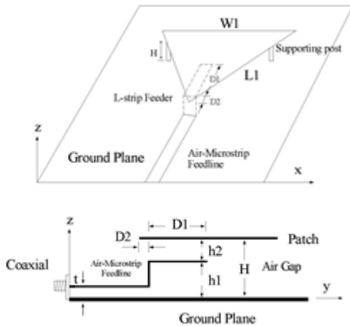
그림 6. L-스트립 삼각형 패치 안테나 Fig. 6. L-strip-fed triangular patch antenna.
