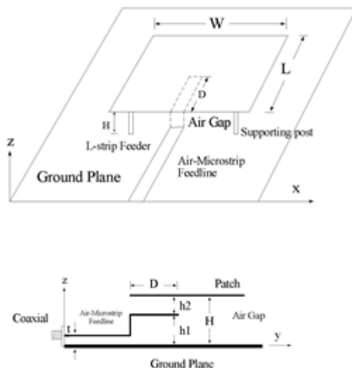
그림 2. L-스트립 사각형 패치 안테나 Fig. 2. L-strip-fed rectangular patch antenna.
