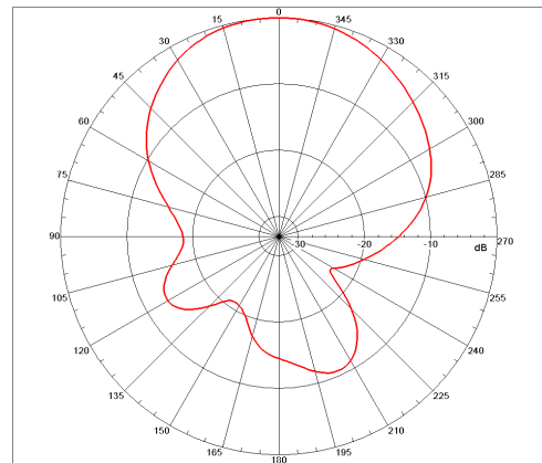
(b) E-plane
