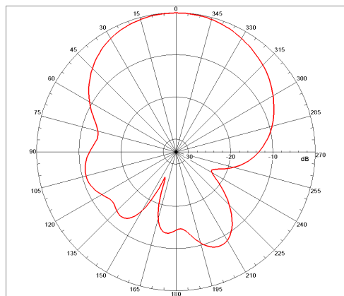
(b) E-plane
