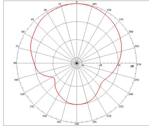
(a) H-plane
