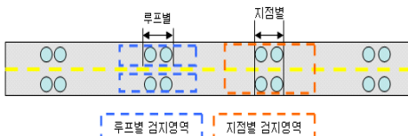
그림 2. 차량검지기 공간적 대상범위(원시자료) Fig. 2. Detective spatial scopes on vehicle detector(Source data)
