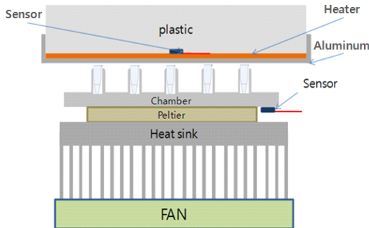
그림 2. 부속 하드웨어 장비 구성도 Fig. 2. Configuration of Hardware Components
