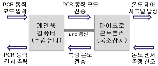
그림 1. 주컴퓨터-국소장치 구조 Fig. 1. Host-Local Structure
