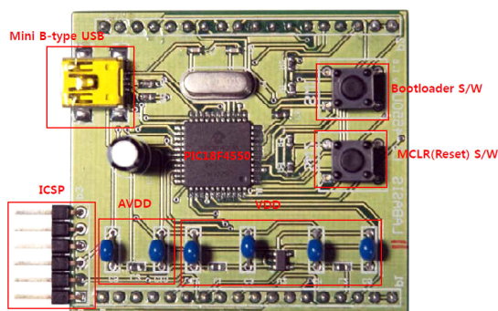
그림 6. 제작된 제어 보드 Fig. 6. Prototype Control Board
