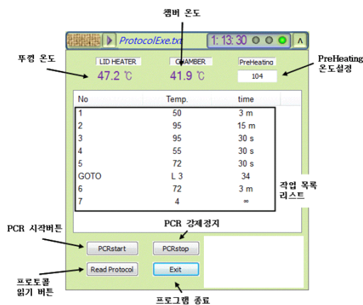
그림 5. 주컴퓨터의 그래픽 인터페이스 프로그램 Fig. 5. Graphic Interface Program in Host Computer
