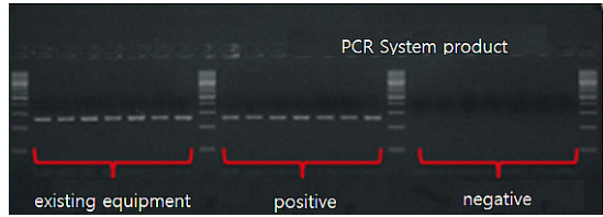
그림 8. PCR 증폭 분석 결과 Fig. 8. Analysis Result of PCR Amplification
