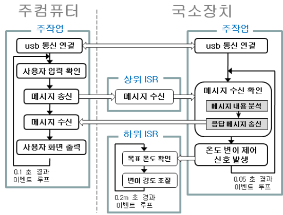
그림 3. 입출력 인터페이스 및 펌웨어 동작 흐름도 Fig. 3. Operation Flows of IO Interface and Firmware
