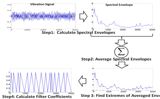
그림 3. 스펙트럴 엔벨로프 기반 필터 설계 Fig. 3. Filter design based on spectral envelope
