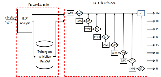
그림 2. 제안한 고장 분류 시스템 Fig. 2. The proposed fault classification system
