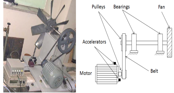
그림 5. 유도전동기의 고장 검출을 위한 실험 시스템 Fig. 5. Experiment system for the fault detection of induction motors
