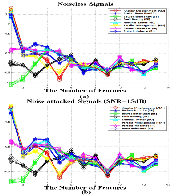
그림 4. SECC에 의해 추출된 특징 벡터 Fig. 4. Feature vectors extracted by SECC
