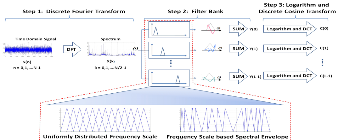
그림 1. 캡스트럼 계수 계산을 위한 단계 Fig. 1. The procedure for the cepstral coefficients computation
