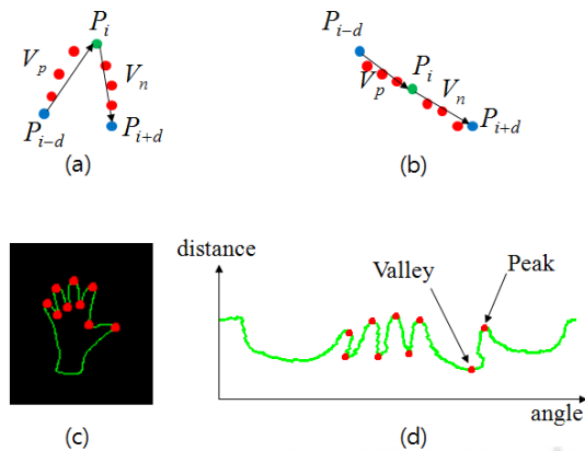
그림 7. 관심점 추출 Fig. 7. Interest point extract
