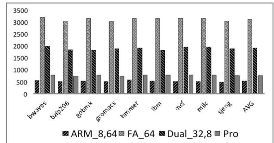
그림 4. 에너지 소비(J) Fig. 4. Energy consumption(J)
