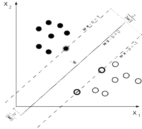
그림 5. SVM 클래스 분류 Fig. 5. SVM class classification
