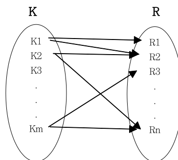
그림 5. 키워드-리소스 매핑을 모델링하는 이분 그래프. Fig. 5. Bipartite graph modeling Keywords to Resources
