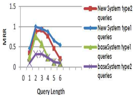
그림 9. MRR-질의 길이 플롯 Fig. 9. MRR-Query Length Plot
