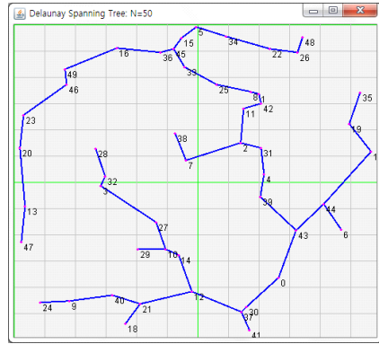
그림 11. 입력노드에 대한 들로네 삼각망 기반 유클리드 최소신장트리 Fig.11. Euclidean Minimum Spanning Tree based on Delaunay Triangulation for Input Nodes
