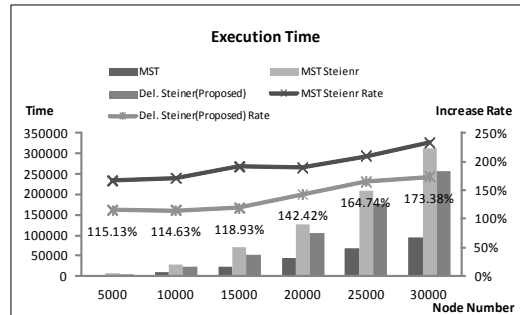
그림 14. 입력노드 수 변화에 따른 트리 생성 시간 Fig.14. Execution Time by Input Node Number for Tree Formation
