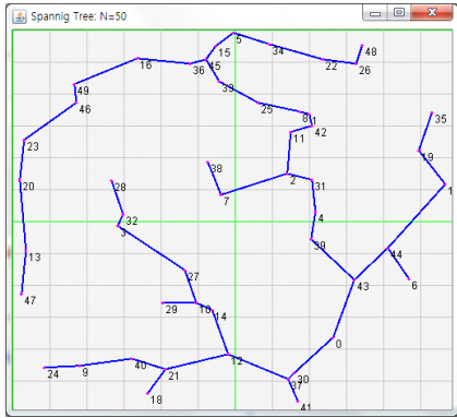
그림 8. 입력노드에 대한 Prim의 알고리즘 기반 유클리드 최소신장트리 Fig.8. Euclidean Minimum Spanning Tree based on Prim's Algorithm for Input Nodes
