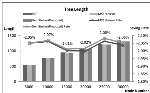
그림 13. 입력노드 수에 따른 생성된 트리 길이 Fig.13. Tree Length by Input Node Number
