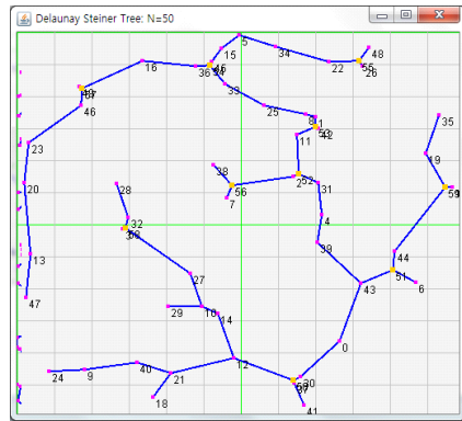
그림 12. 제안방법의 유클리드 스타이너최소트리 Fig.12. Proposed Euclidean Steiner Minimum Tree
