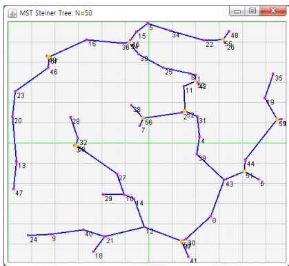
그림 9. 최소신장트리기반 유클리드 스타이너 최소트리 Fig.9. Euclidean Steiner Minimum Tree based on Minimum Spanning Tree for Input Nodes
