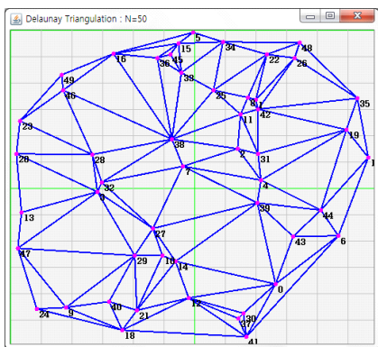
그림 10. 50개 입력노드의 들로네 삼각망 Fig.10. Delaunay Triangulation of 50 Input Nodes
