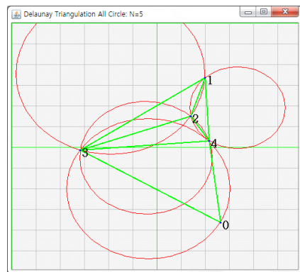
그림 4. 새로운 삼각망의 외접원 집합 Fig.4. Circumcircle Set of New Triangulation
