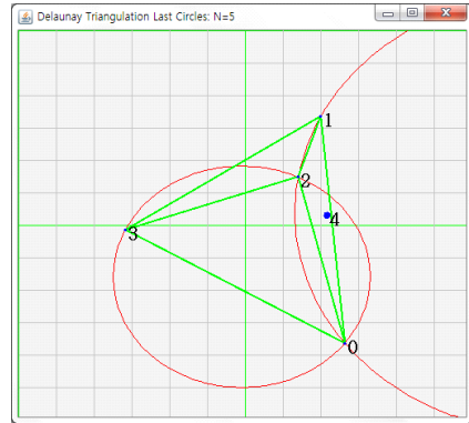
그림 2. 새로운 정점 4의 입력 Fig.2 Insert of Vertex 4
