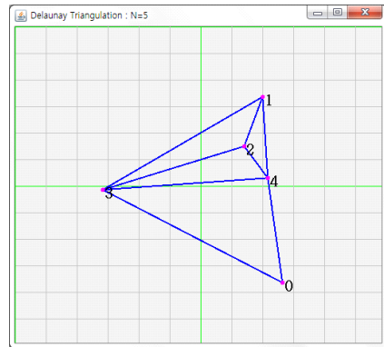
그림 3. 새로운 삼각망의 구성 Fig.3. Formation of New Triangulation
