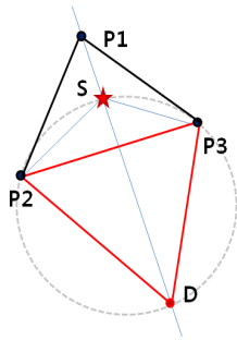
그림 5. 스타이너 포인트 생성 Fig.5. Locating of Steiner Point
