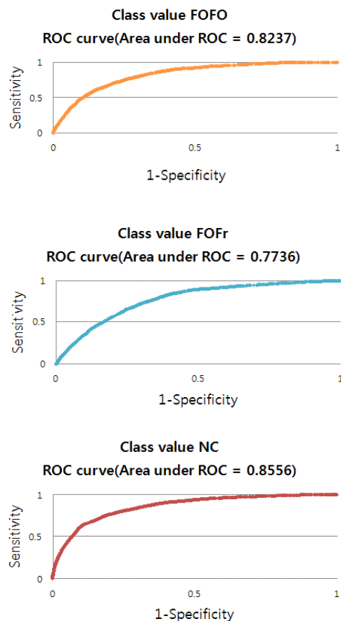
그림 3. Decision Table 알고리즘의 클래스별 ROC curve
