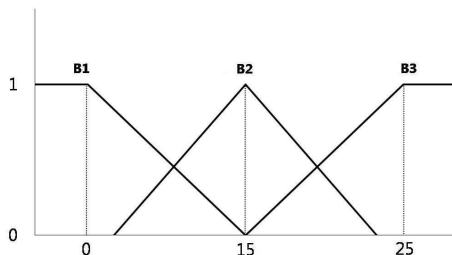
그림 8. 지속기간에 대한 퍼지 소속 함수 Fig. 8. Membership Function for Duration
