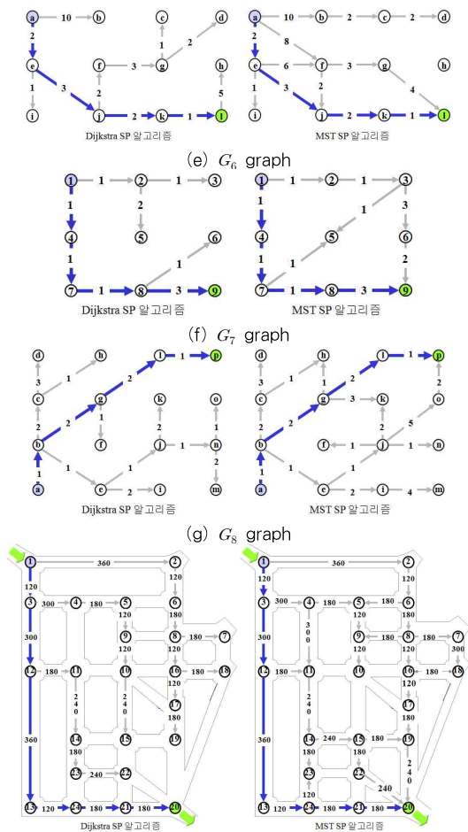
(e) G_6 graph (f) G_7 graph (g) G_8 graph (h) G_9 graph 그림 6. 최단경로 Fig. 6. Shortest path
