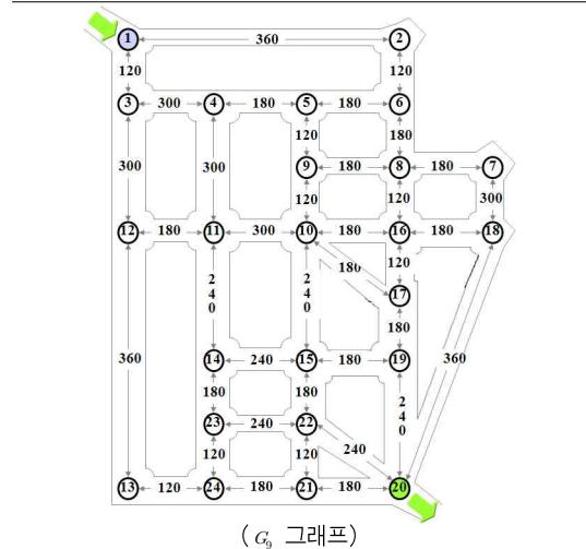
그림 5. 실험에 적용된 그래프 Fig. 5. Experimental graph
