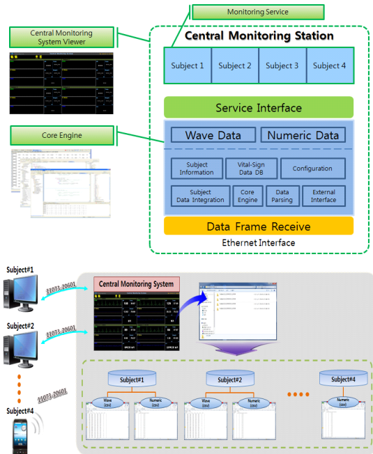
그림 8. 다중 생체신호 중앙 모니터링 시스템 소프트웨어의 구조 Fig. 8. Multiple Bio-Signal Central Monitoring System Software Architecture
