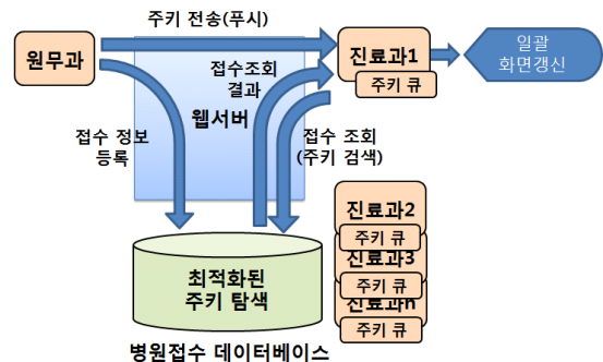
그림 1-2. 주키전송에 의한 일괄처리 접수시스템 Fig. 1-2. Batch Reception System using Primary Key Transmission
