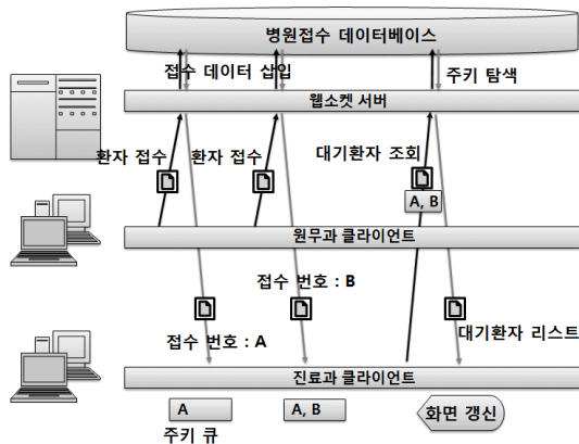
그림 3-2. 주키전송 일괄처리 접수시스템 흐름도 Fig. 3-2. Batch Reception System Flowchart by Transmitting Primary Key
