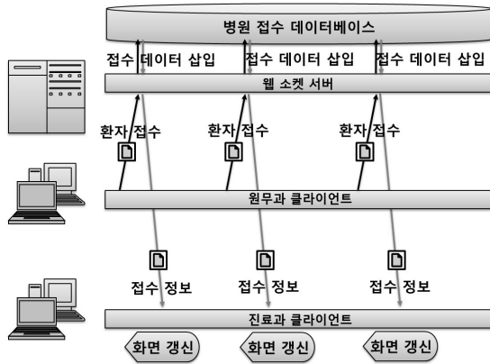
그림 3-4. 접수정보전송 실시간 접수시스템 흐름도 Fig. 3-4. Real Time Reception System Flowchart by Transmitting Reception Information
