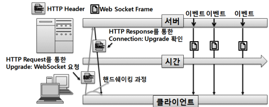
그림 2-6. 웹소켓 기술 Fig. 2-6. Web Socket Technology
