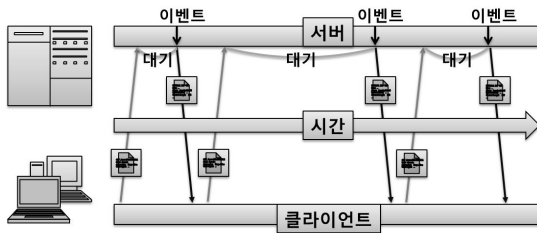
그림 2-5. Long-Polling 기법 Fig. 2-5. Long-Polling Method
