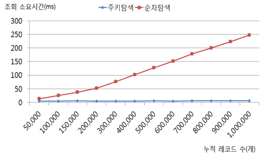
그림 4-9. 주기탐색과 순차탐색 시간 비교 Fig. 4-9. Time Comparison between Primary Key and Sequential Searches
