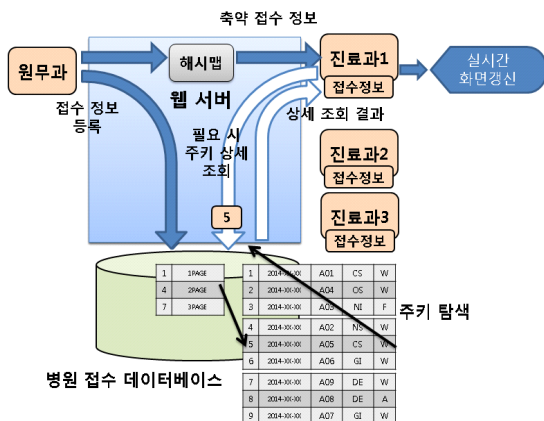
그림 3-5. 접수정보전송 실시간 접수시스템 구조도 Fig. 3-5. Real Time Reception System Structure by Transmitting Reception Information
