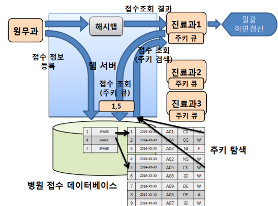
그림 3-3. 주키전송 일괄처리 접수시스템 구조도 Fig. 3-3. Batch Reception System Structure by Transmitting Primary Key
