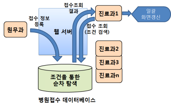
그림 1-1. 순차탐색에 의한 일괄처리 접수시스템 Fig. 1-1. Batch Reception System using Sequential Search
