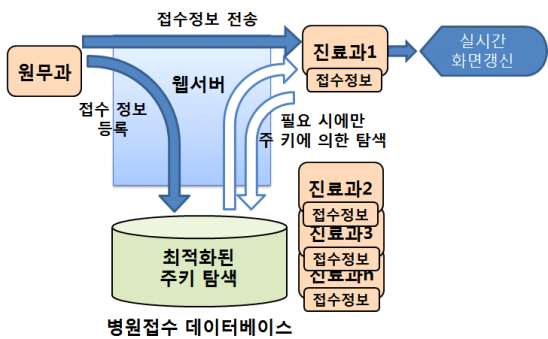
그림 1-3. 접수정보전송에 의한 실시간 접수시스템 Fig. 1-3. Real Time Reception System by Transmitting Reception Information
