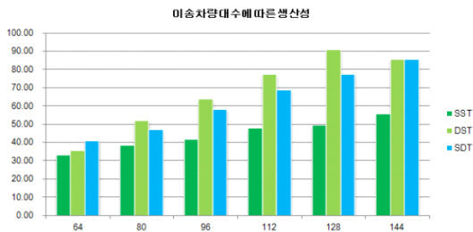
그림 7. 이송차량 대수에 따른 컨테이너 생산성 Fig. 7. The Productivity of Container according to Transport vehicle number
