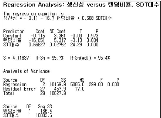
그림 11. 이송차량이 SDT 일 때의 회귀분석 결과 Fig. 11. Regression analysis of SDT
