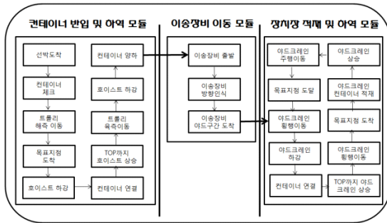
그림 3. 시물레이션 모듈 구조 Fig. 3. Structure of Simulation module
