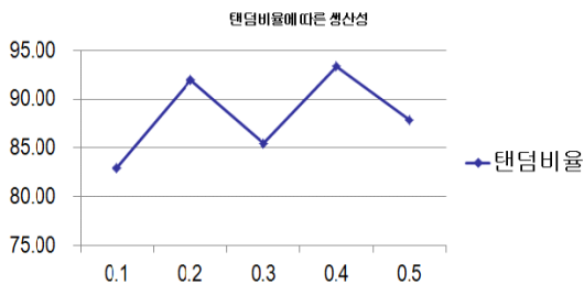
그림 6. 탠덤비율에 따른 컨테이너 생산성 Fig. 6. The Productivity of Container according to Tandem ratio
