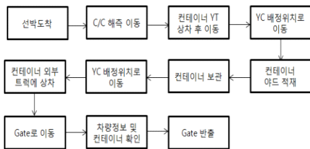
그림 2. 컨테이너터미널의 수입 프로세스 Fig. 2. Import process of Container terminal
