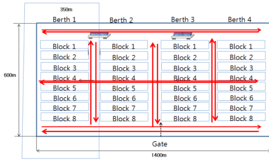
그림 1. 컨테이너터미널의 configuration Fig. 1. Configuration of Container terminal
