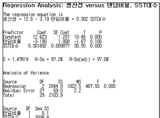
그림 10. 이송차량이 DST 일 때의 회귀분석 결과 Fig. 10. Regression analysis of DST
