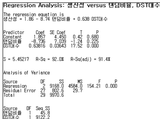
그림 9. 이송차량이 SST 일 때의 회귀분석 결과 Fig. 9. Regression analysis of SST
