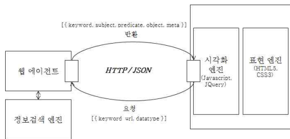
Fig. 18. A Flow of Web Interface
