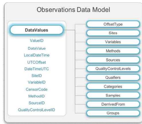
Fig. 4. CUAHSI ODM Overview
