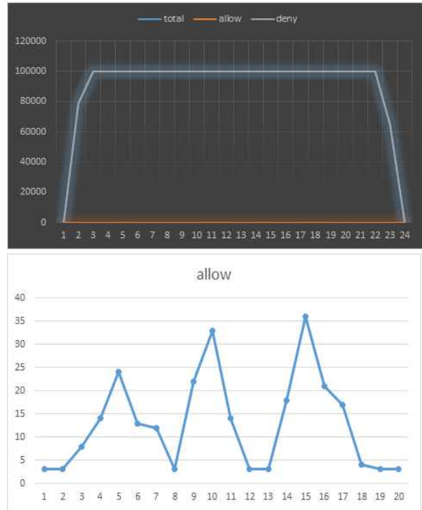
Fig. 8. Packet status
