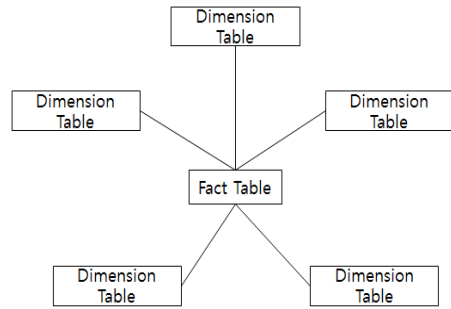
Fig. 1. Star Schema
