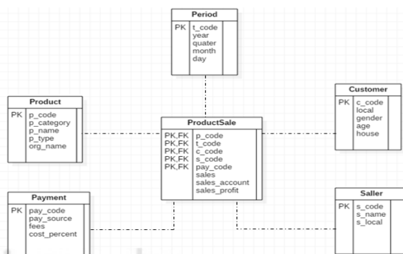
Fig. 7. Physical Star Schema
