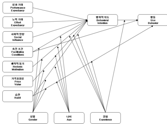
Fig. 1. UTAUT2
