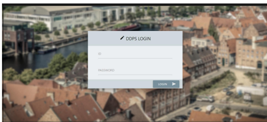
Fig. 6. Login screen
