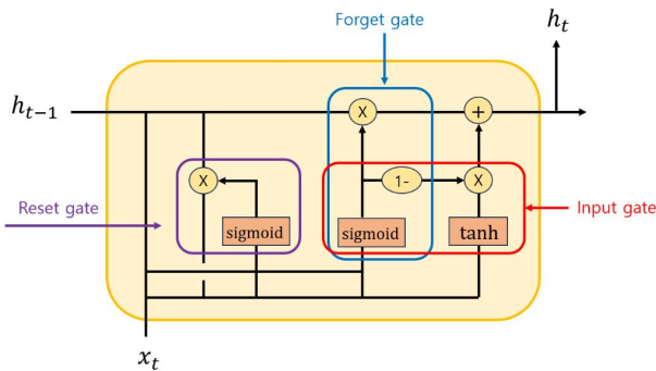
Fig. 1. GRU Network
