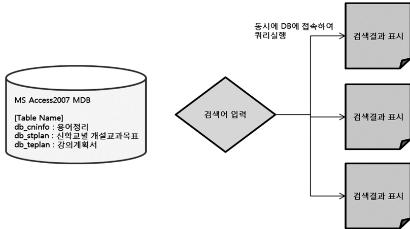
〈그림 2〉 키워드 검색시스템의 로직 진행순서
