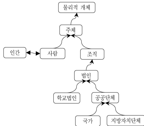
<그림 4> 주체의 포함 관계
