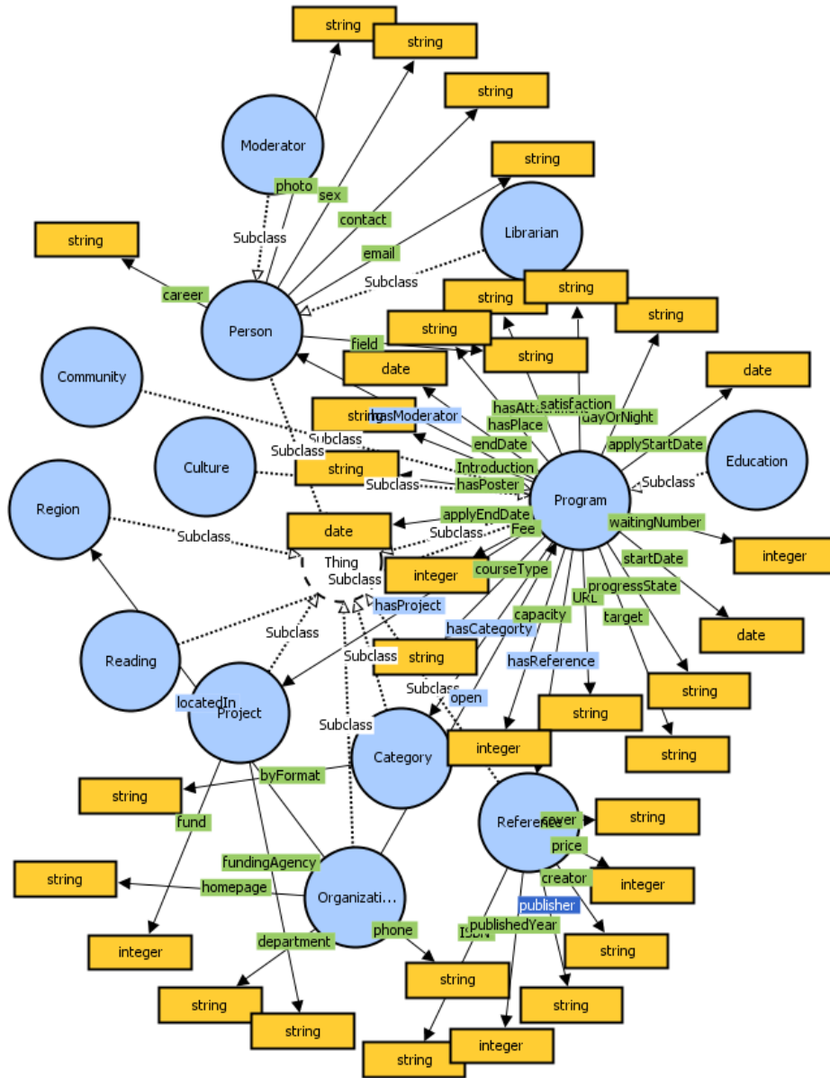
〈그림 4〉 데이터 모델링 결과 시각화 예시
