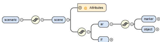
[Fig. 6] AR-SML Schema
