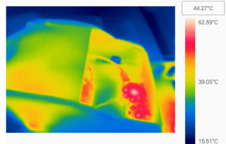
[Fig. 3] Thermal Camera Screen
