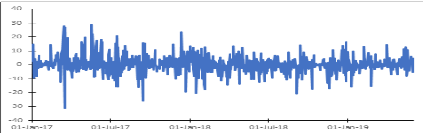
(b) Ethereum
