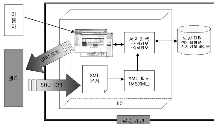
〈그림 4〉 로컬기관 시스템 구성도
