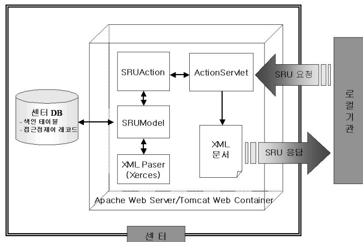
〈그림 3〉 접근점제어 센터 시스템 구성도
