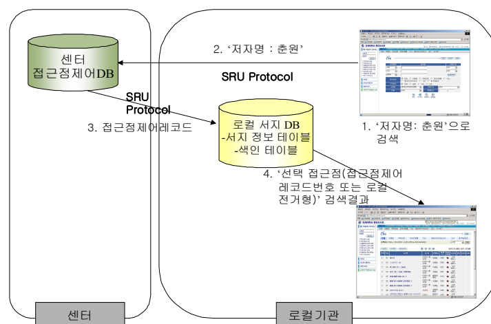
<그림 2> 접근점제어 시스템의 OPAC 검색 개념도
