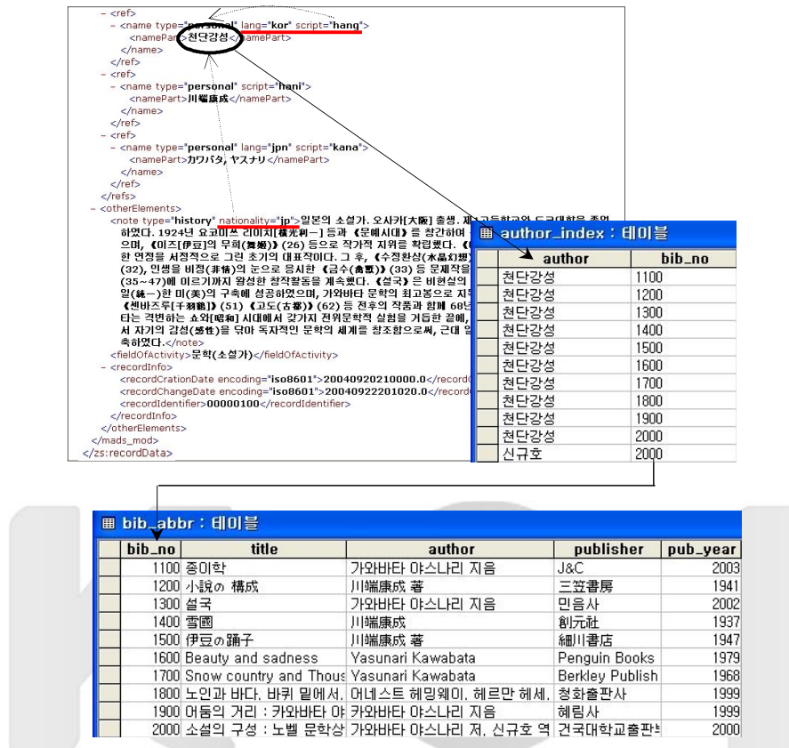
〈그림 6〉 로컬기관 저자 연계(방식2)
