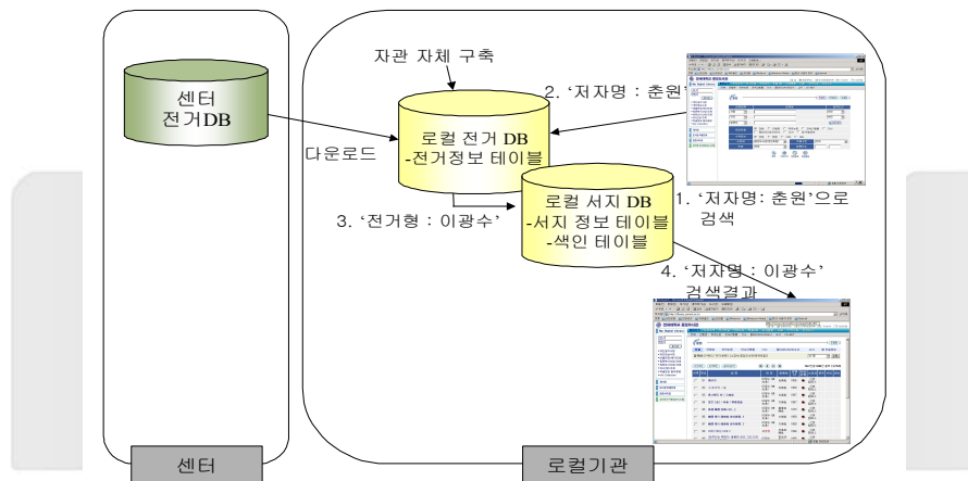
<그림 1> 기존 선거제어 시스템의 OPAC 검색 개념도
