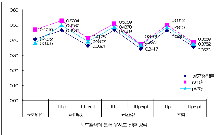
그림 3. 노드검색의 성능 비교
