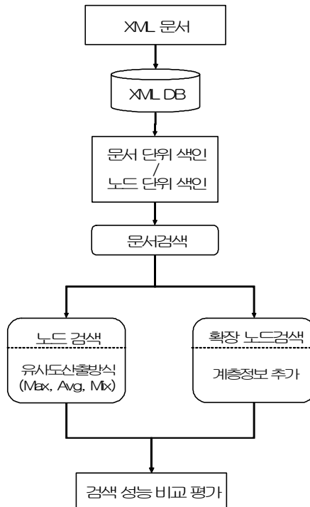
그림 1. 노드검색 실험과정
