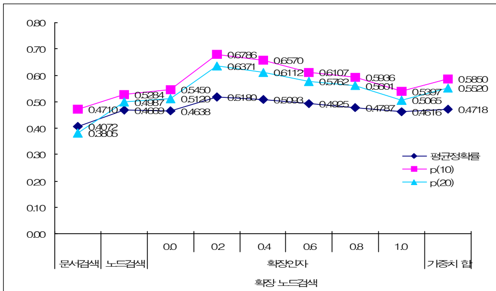
그림 4. 확장 노드검색의 성능 비교
