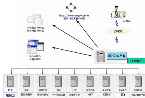
<그림 1> 국가지식포털 연계 구조
