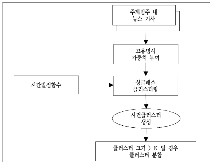
<그림 3> 사건 클러스터 생성 개요
