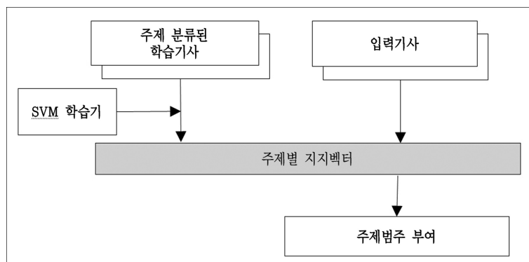
〈그림 2〉 주제범주 자동분류 개요
