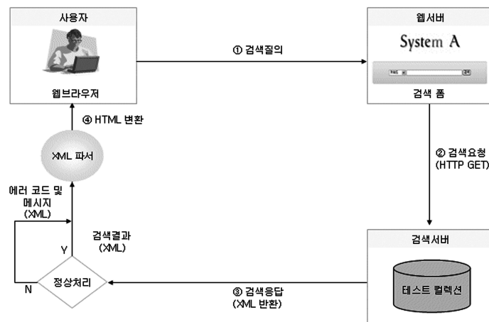
<그림 3> 시스템 A의 구성도
