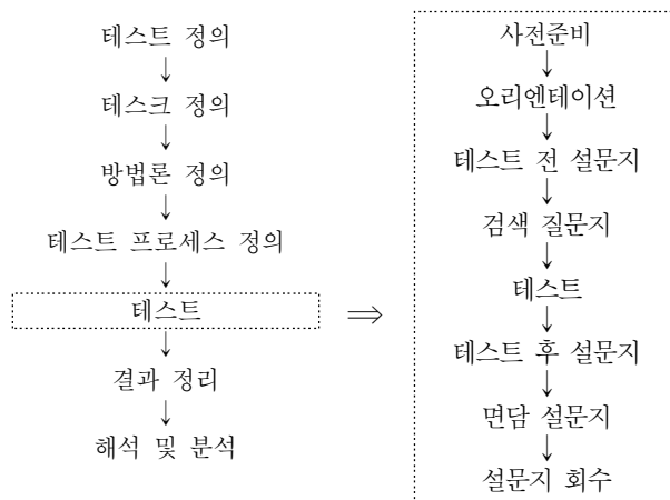
<그림 2> 사용성 평가 및 평가자료 수집 절차
