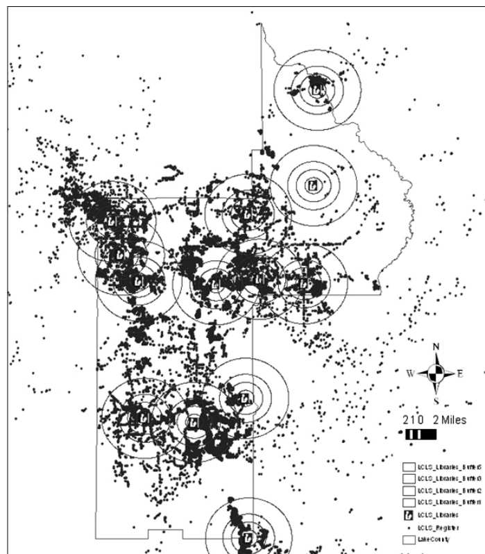
<그림 4> 1, 3, 5마일 버퍼 결과
