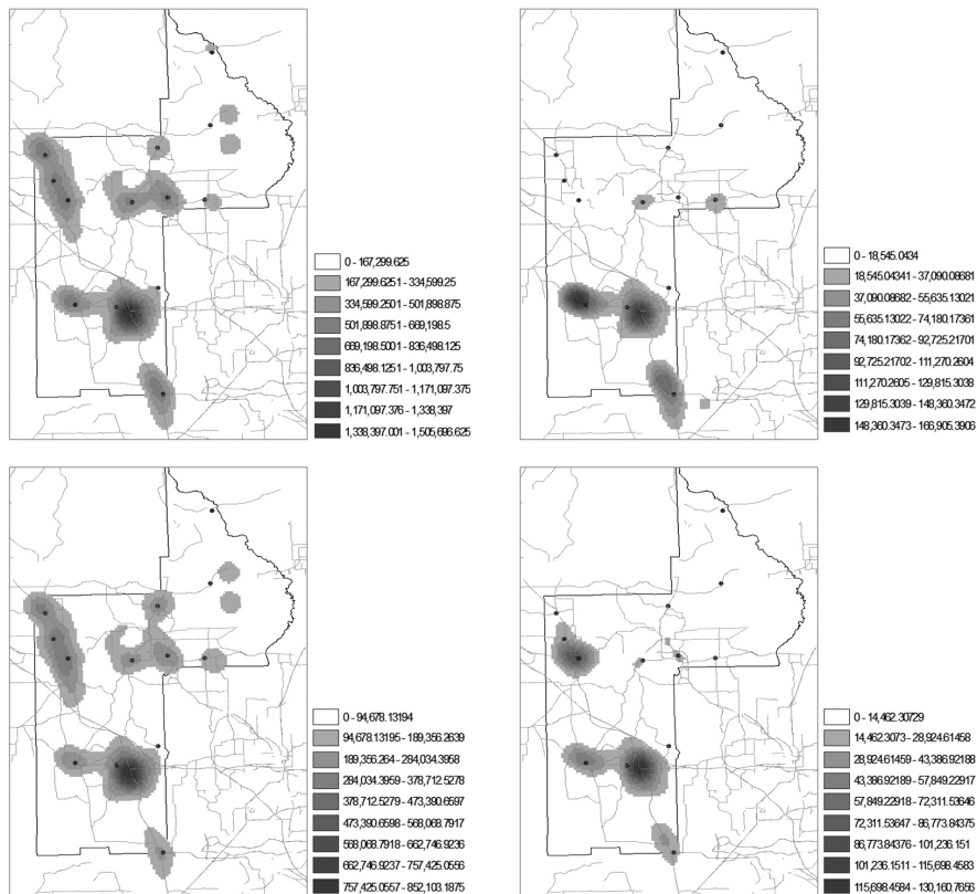
〈그림 3〉 인종에 따른 밀집도 분석 결과
