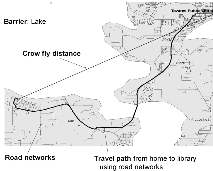
〈그림 5〉 유클리디언 함수와 도로망을 이용한 거리측정 방식 비교
