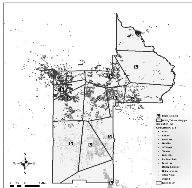
〈그림 2〉 Lake 카운티 공공도서관의 서비스 구역 설정
