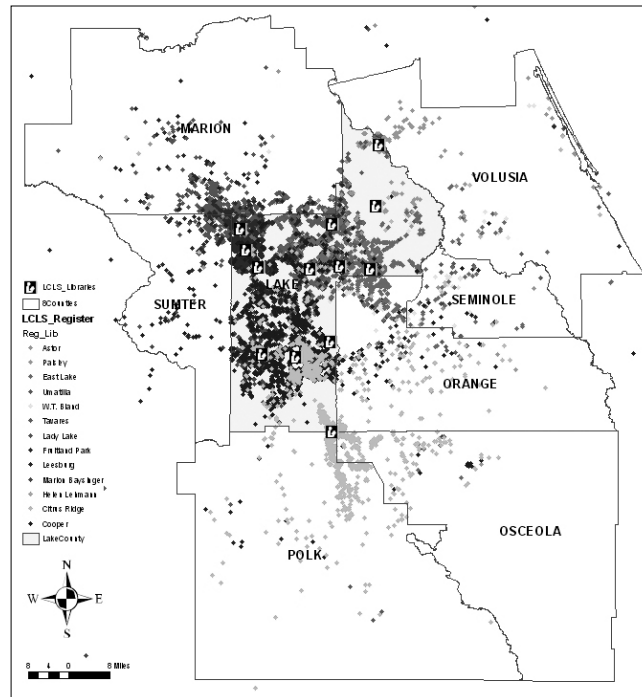
〈그림 1〉 Lake County 공공도서관과 이용자 위치
