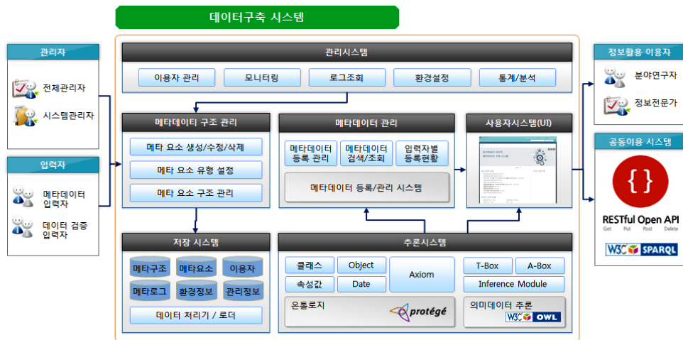
〈그림 2〉 시스템 구성도
