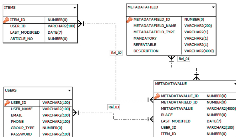
〈그림 3〉 KMD DB의 핵심 테이블 ERD(Entity-Relationship Diagram)
