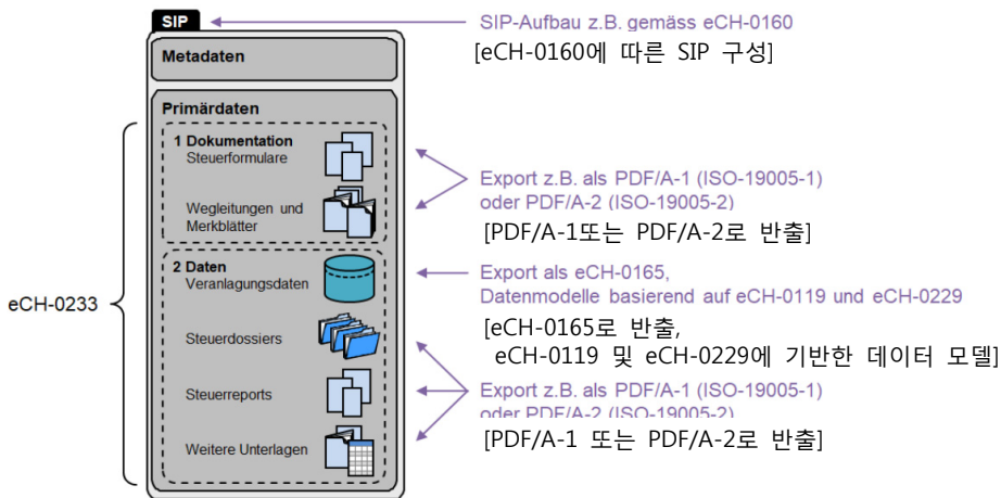
〈그림 3〉 eCH-0233 개요 출처: eCH-0233 (2019)
