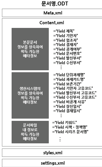
〈그림 1〉 공문서 ODT Content.xml에서 추출 가능한 메타데이터
