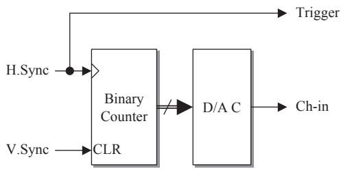
그림 3. 수직신호 발생 원리 Fig. 3. Principle of vertical signal generation
