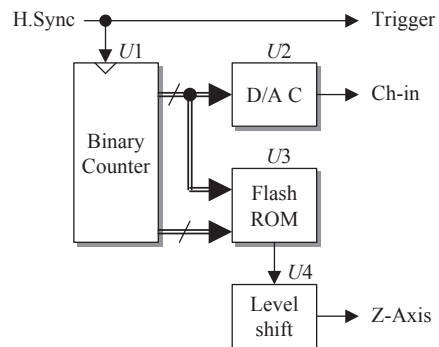
그림 4. 실험회로의 블록도 Fig. 4. Block diagram of experimental circuit
