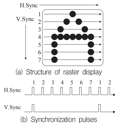
그림 1. 라스터 디스플레이의 신호들 Fig. 1. Signals of raster display
