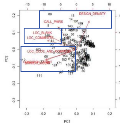
그림 9. 2차원 그래프(차원수=3)
