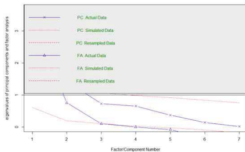
그림 6. 스크리 그래프
