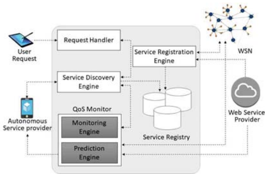
그림 2. SOA기반 IoT 미들웨어 구조 Fig. 2. SOA based IoT middleware architecture
