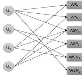
그림 5. 호출관계 그래프
