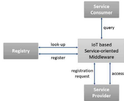
그림 1. 사물기반 SOA Fig. 1. Thing-based SOA
