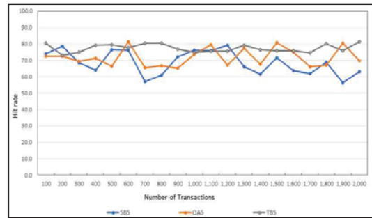
그림 6. 적중률 비교
