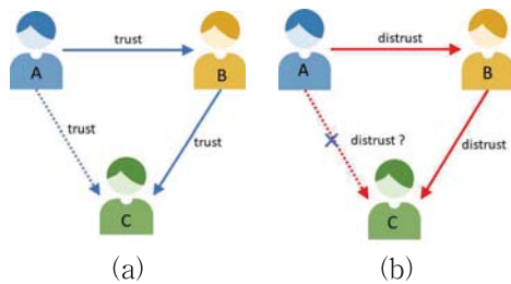
그림 4. 신뢰의 전이
