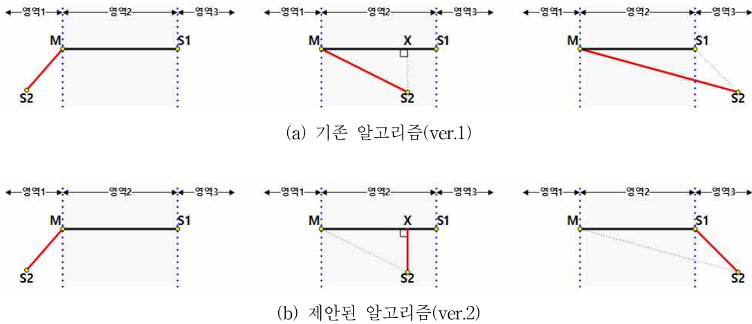
그림 1. 기존 알고리즘(ver.1)과 제안된 알고리즘(ver.2) 동작 Fig. 1. Operations of ver.1 and ver.2 algorithms
