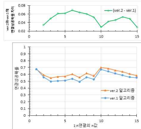
그림 4. 8x8 2차원 스위치 구조의 1:n 연결성공확률 Fig. 4. 1:n connection success probability in 8x8 2-dimensional switch architecture
