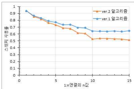
그림 6. 8x8 2차원 스위치 구조에서 1:n 연결의 스위치 사용률
