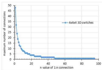
그림 3. 4x4x4 3차원 스위치 구조의 1:n 연결 최대개수
