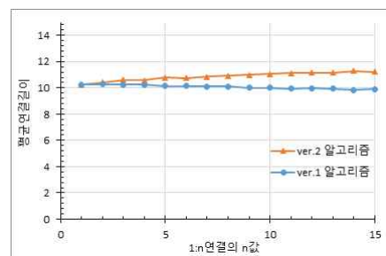
그림 5. 8x8 2차원 스위치 구조에서 1:n 연결의 평균경로길이 Fig. 5. Average path length of 1:n connection in 8x8 2-dimensional switch architecture
