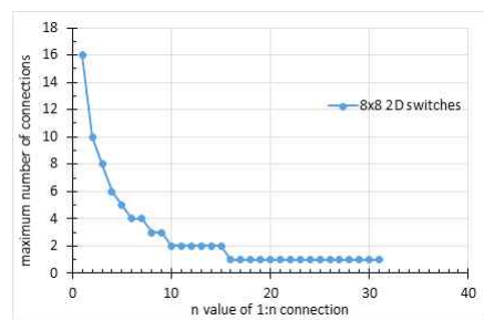
그림 2. 8x8 2차원 스위치 구조의 1:n 연결 최대개수 Fig. 2. Maximum number of 1:n connections in 8x8 2-dimensional switch architecture
